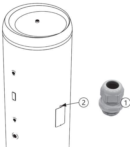
El-kobling, skjematisk
