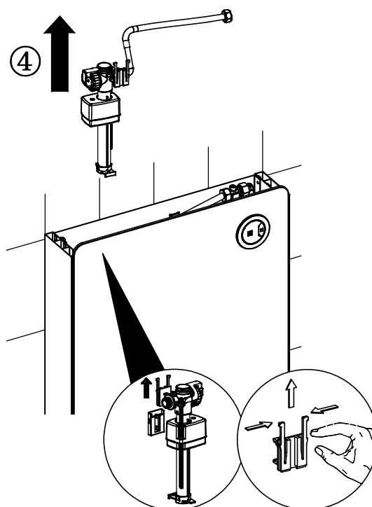
Løsne innløpsventilen
