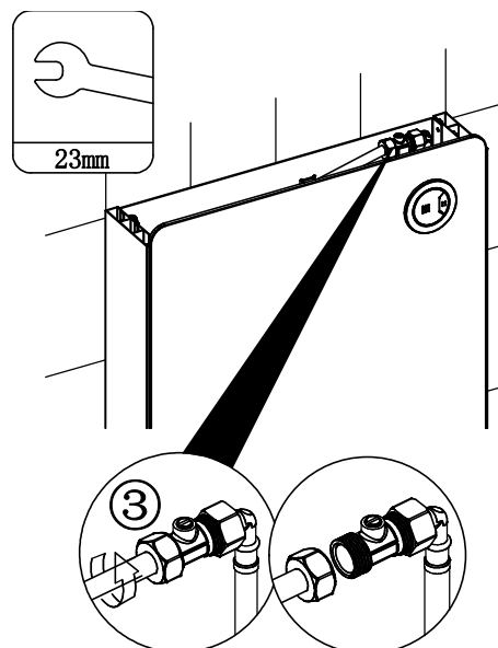
Koble fra slange og ventil
