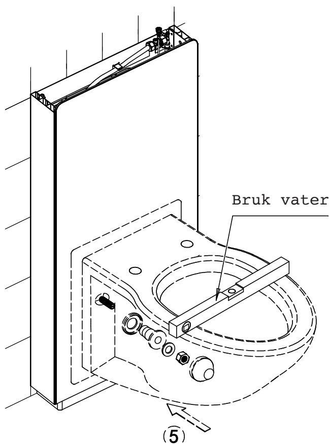
Montér toalettet
