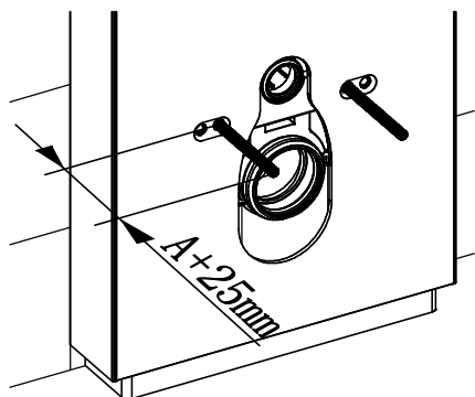
Fest sisternerammen
