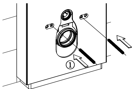
Fest sisternerammen
