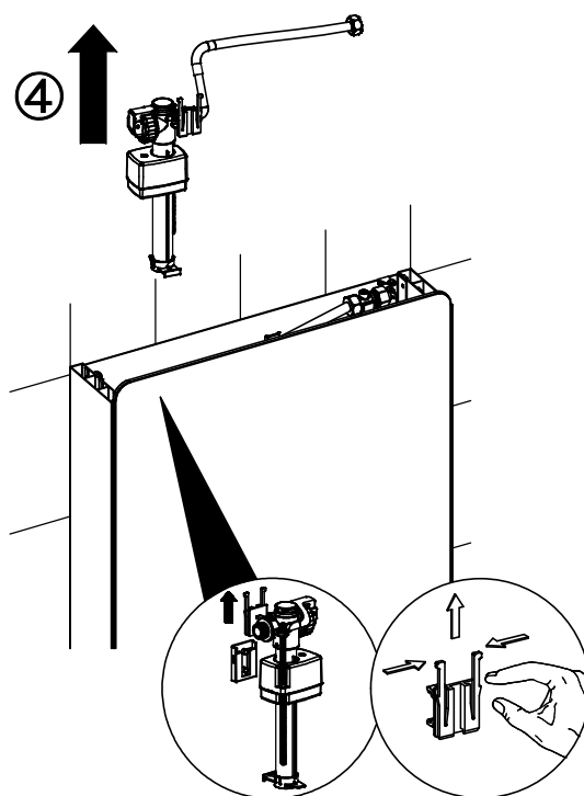
Løsne innløpsventilen
