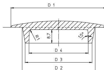
Tubman Universalpropp i gummi.
