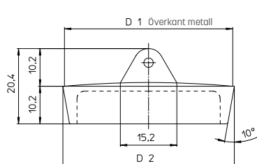
Tubman Gummipropp, vissa storlekar finns även med förkromad lös topp.
