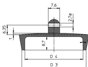
Tubman Gummipropp, vissa storlekar finns även med förkromad lös topp.
