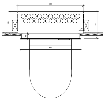
2 UNOPAX BACK DOOR
